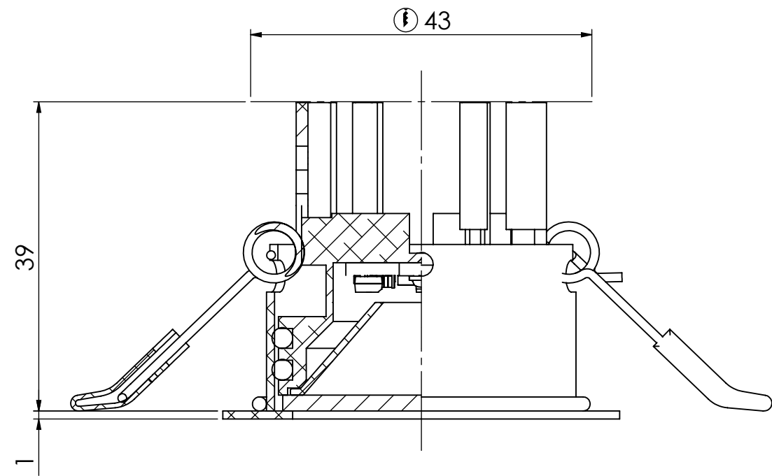
SEZIONE A-A
